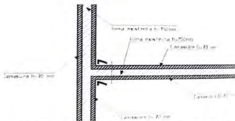
Detaliu 1 - Camasuiri pereti din zidarie pe ambele fete
