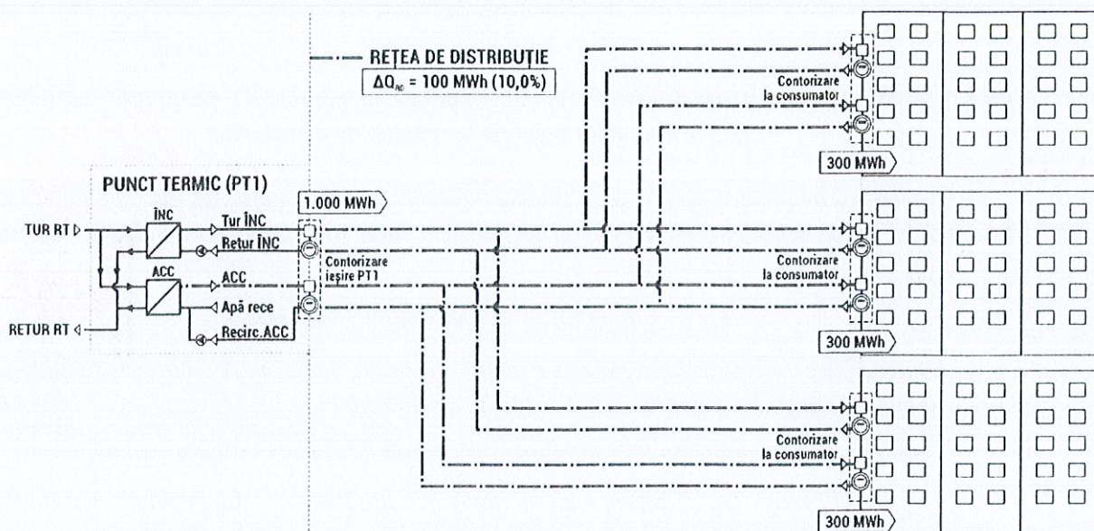
Fig. 8.1. Rețea de distribuție existentă – varianta inițială (de proiect), la momentul t_1
