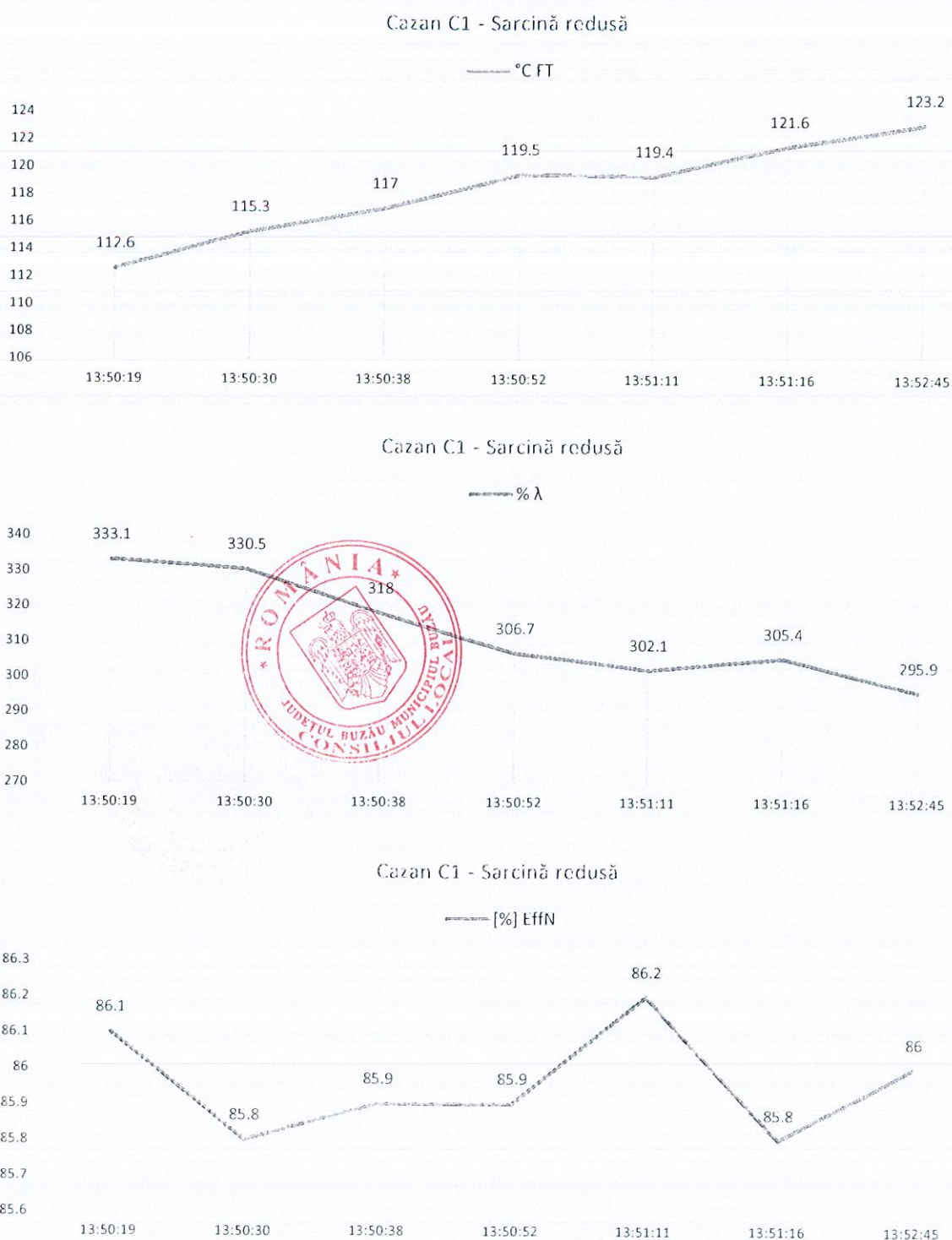
Fig. 6.13. Evoluția valorilor temperaturii gazelor de ardere (°C FT), excesului de aer de ardere (% λ) și a eficienței arderii ([%] EffN) la sarcină redusă, la cazanul C1 – CT Integral
