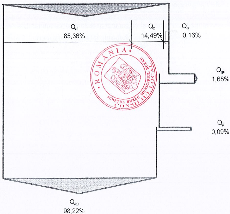
Fig. 6.7. Diagrama Sankey pentru bilanțul real anual al cazanului C2 din CT 5 Micro XIV
