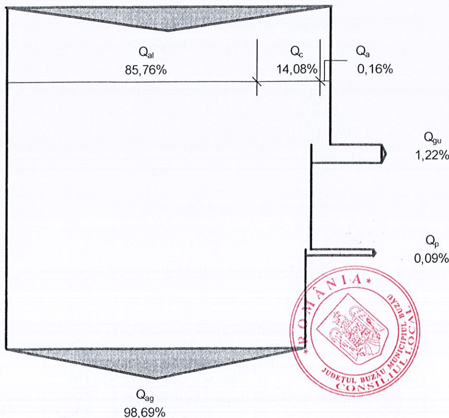
Fig. 6.6. Diagrama Sankey pentru bilanțul real anual al cazanului C1 din CT 5 Micro XIV
