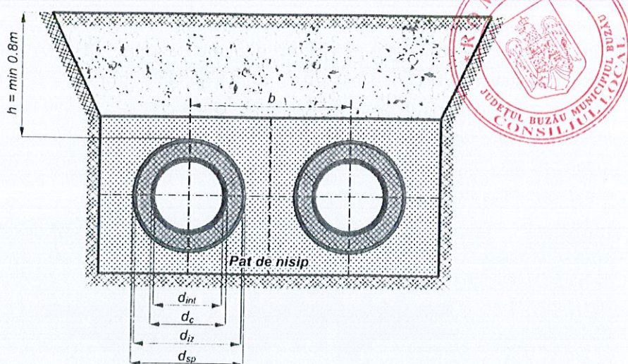
Fig. 5.2. Secțiune transversală de conducte preizolate așezate în pământ
