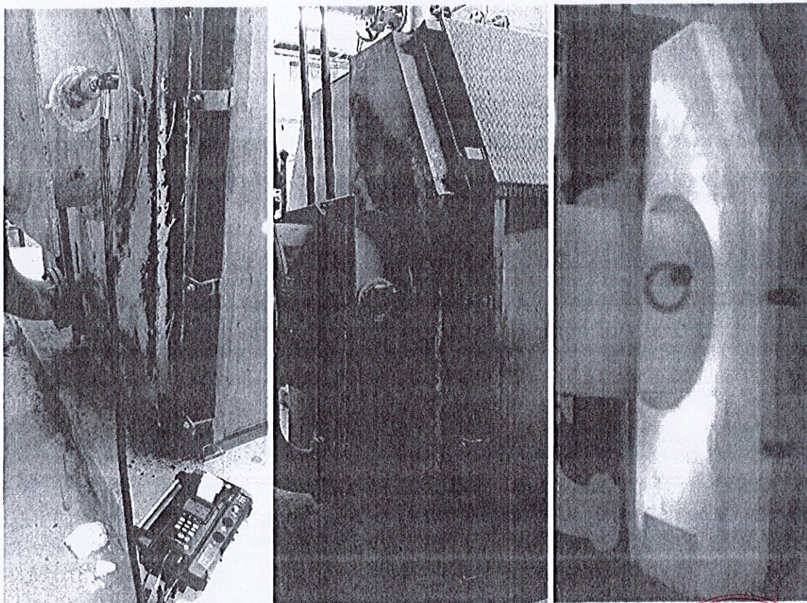
Fig. 6.e. CT4 Dorobanți: analiză gaze de ardere la cazanul HR3-3200, cu analizorul de gaze Testo 300 XXL, respectiv inspecție termografică pentru determinare pierderi de căldură prin pereții cazanului
