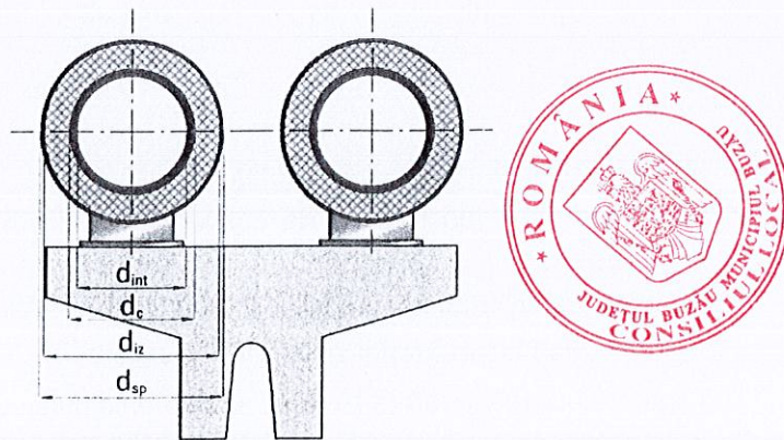
Fig. 5.1. Secțiune transversală de conducte preizolate pozate aerian
