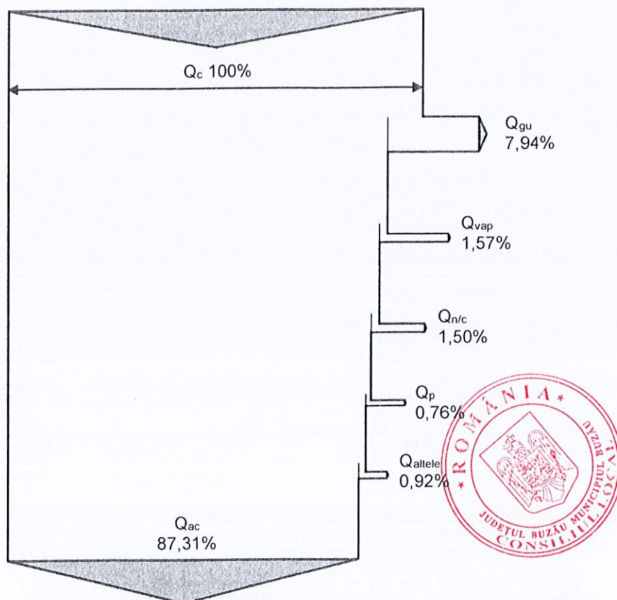
Fig. 6.15. Diagrama Sankey pentru bilanțul real anual pe conturul CT Integral (bilanț de combustibil)
