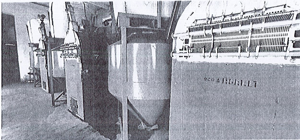
Fig. 6.12. Sub-contur 4: CT Integral, echipată cu 3 cazane ecoHORNET CTP 350 (525 kW fiecare)
