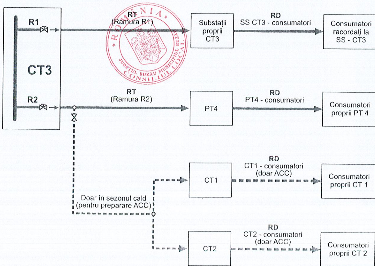
Fig. 6.16. Schema generală de funcționare a CT3 și rețelele de transport și distribuție aferente
