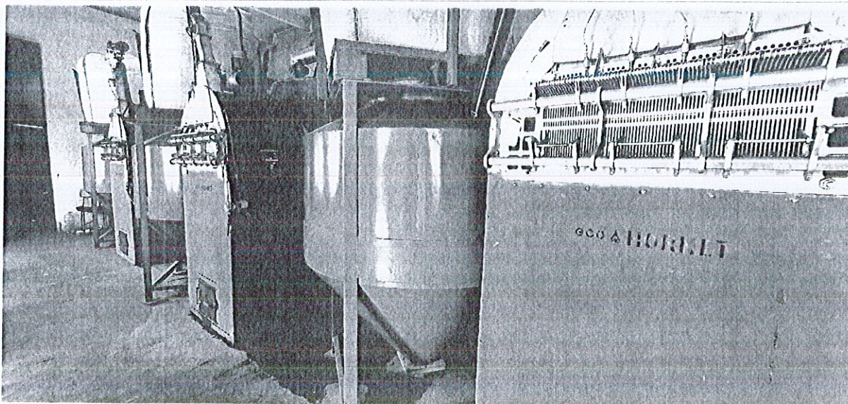
Fig. 2.7. Sub-contur 4: CT Integral, echipată cu 3 cazane ecoHORNET CT 350 (525 kW fiecare)
