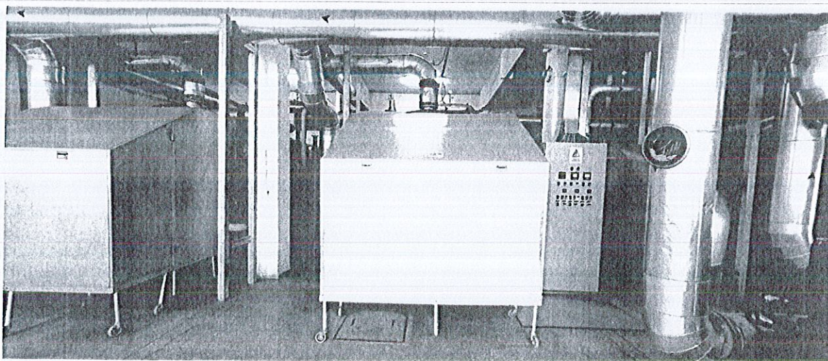
Fig. 6.b. CT3 Micro XIV. Cazane Ygnis Pyronox LD 6000 (stânga) și LR 2150 (dreapta) cu carcase termoizolante pentru reducerea pierderilor de căldură către mediul ambiant prin capacul frontal
