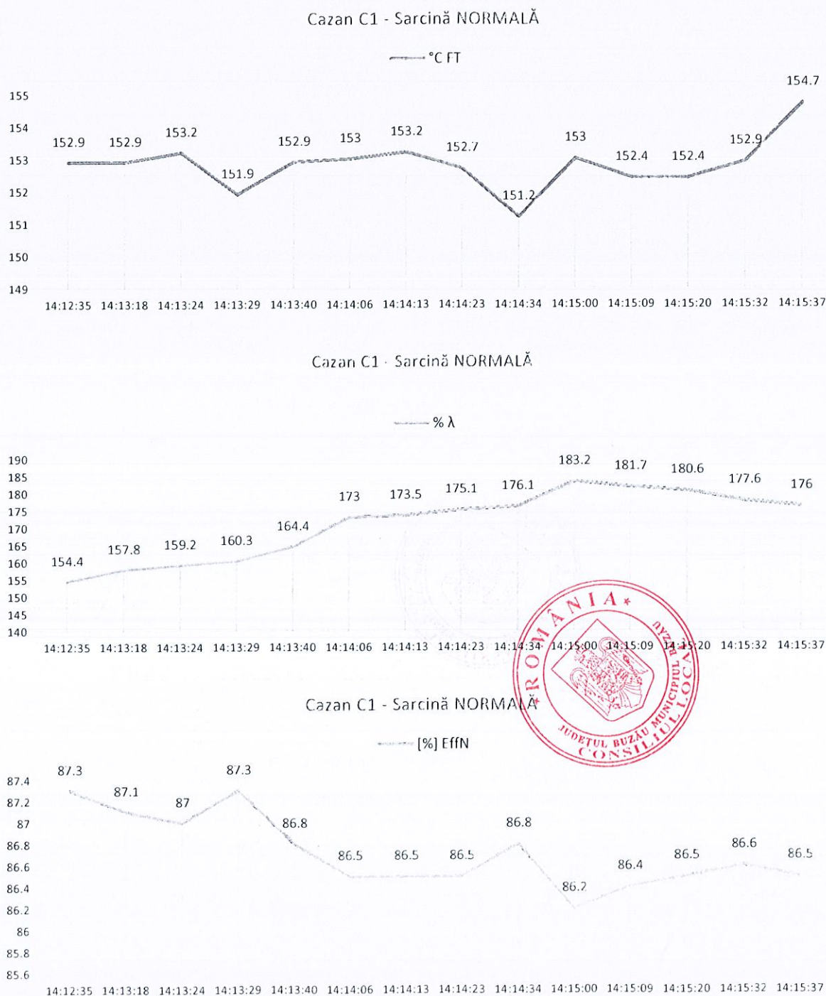
Fig. 6.14. Evoluția valorilor temperaturii gazelor de ardere (°C FT), excesului de aer de ardere (% λ) și a eficienței arderii ([%] EffN) la sarcină nominală, la cazanul C1 – CT Integral
