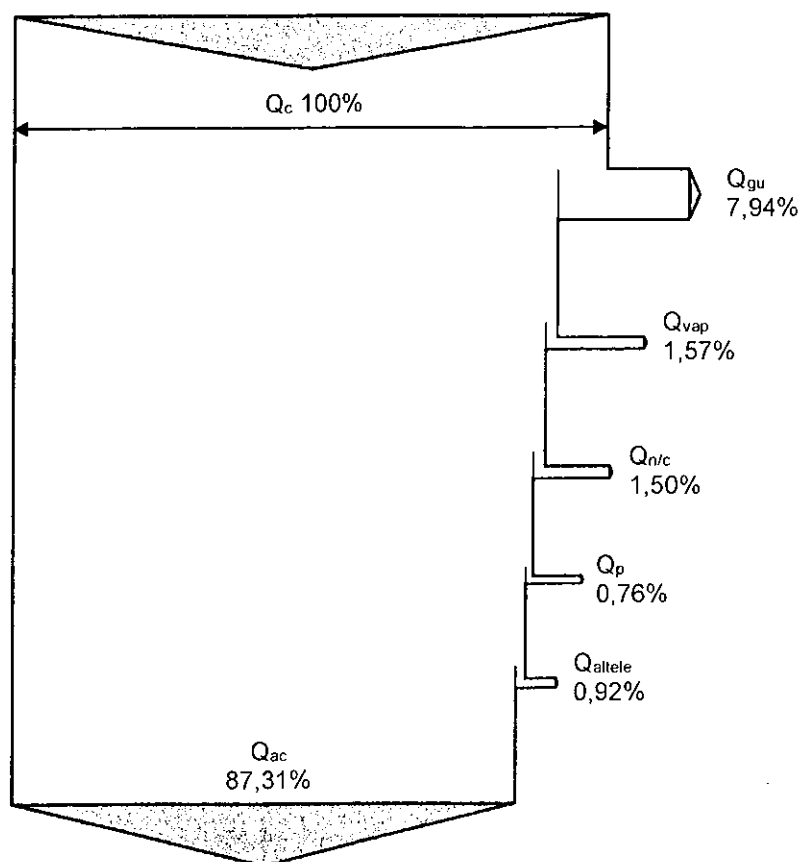
Fig. 6.15. Diagrama Sankey pentru bilanțul real anual pe conturul CT Integral (bilanț de combustibil)
