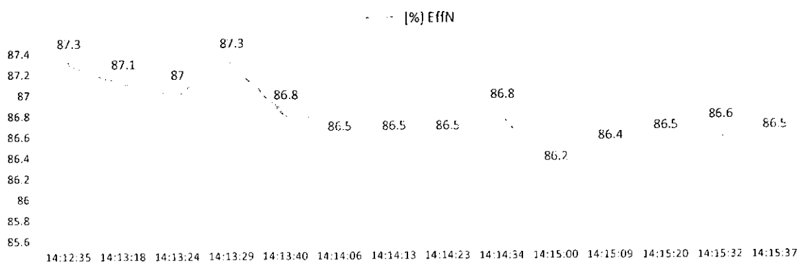
Fig. 6.14. Evoluția valorilor temperaturii gazelor de ardere (°C FT), excesului de aer de ardere (% λ) și a eficienței arderii ([%] EffN) la sarcină normală, la cazanul C1 – CT Integral
