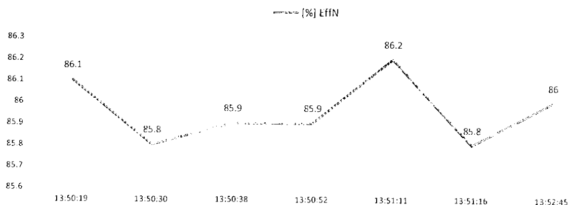
Fig. 6.13. Evoluția valorilor temperaturii gazelor de ardere (°C FT), excesului de aer de ardere (% λ) și a eficienței arderii ([%] EffN) la sarcină redusă, la cazanul C1 – CT Integral
