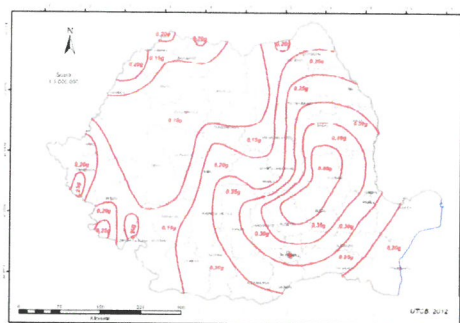
Figura 3.1 România - Zonarea valorilor de vârf ale accelerației terenului pentru proiectare a.c. IMR = 225 ani și 20% probabilitate de depășire în 50 de ani
