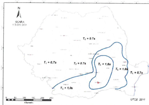
Figura 3.2 Zonarea terenurilor României în termeni de perioada de control (cota), T_c a spectrului de răspuns
