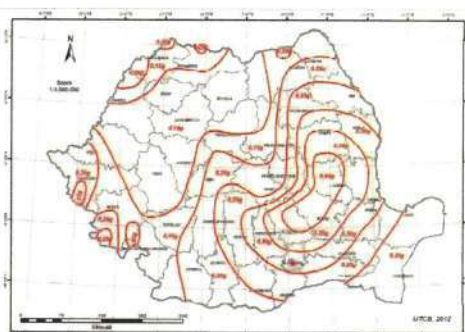
Figura A1 România - Zona de valori de vârf ale accelerației terenului pentru proiectare a_g cu DMR = 225 ani și 20% probabilitate de depășire în 50 de ani
