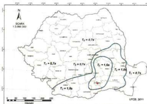
Figura A2 Zona de teritoriul României în termeni de perioada de colț T_c a spectrului de răspuns
