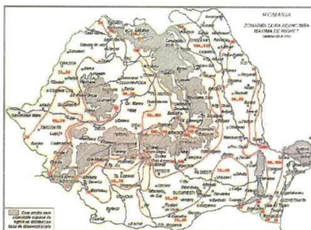
ANEXA 9 - Zona de teritoriul României după adâncimea de îngheț, conform STAS 6054/77, „Adâncimi maxime de îngheț”
