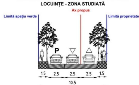
PROFIL PROPUȘ STRADA PROPUȘĂ ÎN CADRUL ANSAMBLULUI DE LOCUINȚE - ZONA STUDIATĂ
