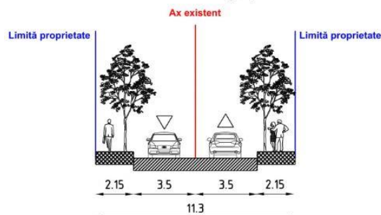
PROFIL PROPUȘ STRADA DEPOZITULUI ȘI STRADA CĂPITAN PURCHEREA LAURENȚIU, SCARA 1:250
