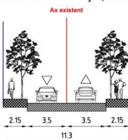
PROFIL PROPUȘ STRADA DEPOZITULUI ȘI STRADA CĂPITAN PURCHEREA LAURENȚIU, SCARA 1:250
